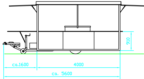
Abwicklung der Brüstungsklappen
